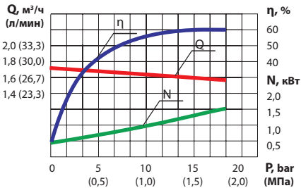
НМШ 2-40-1.6/16
