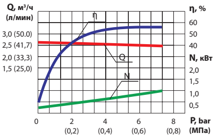
НМШ 5-25-2.5/6
